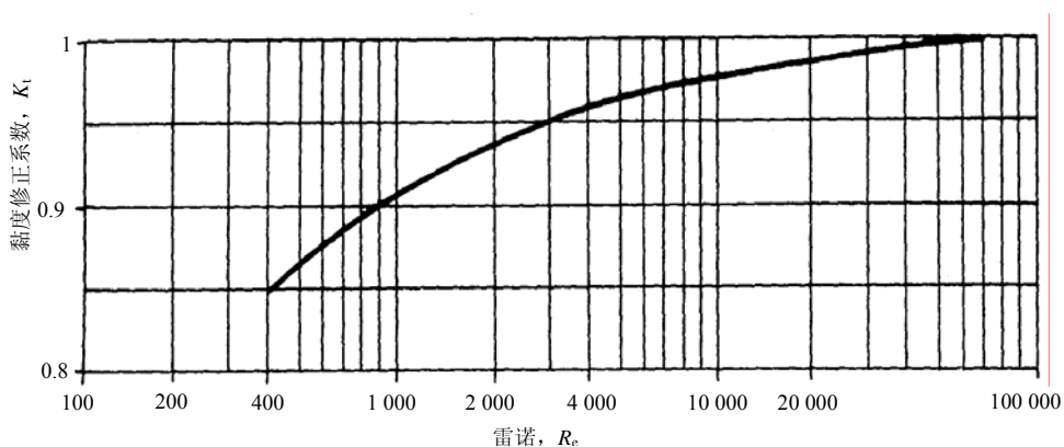
图 D.1 K_r 同 R_e 的关系
