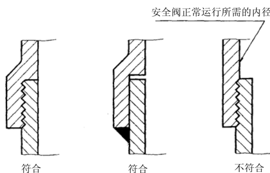
图 1 端部连接的设计
