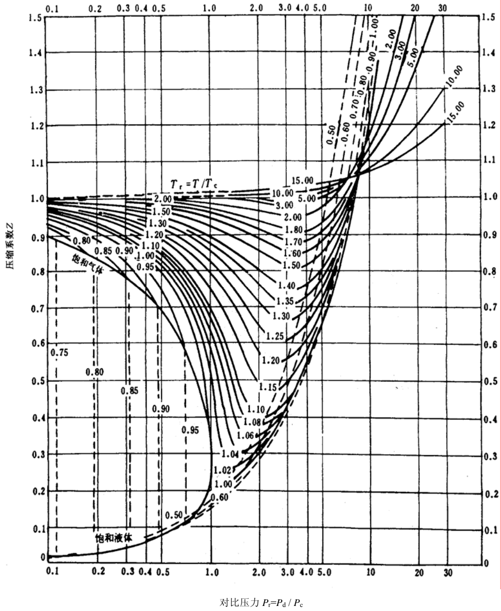
图 B.1 压缩系数 Z 与对比压力 P_r = P_d / P_c 和对比温度 T_r = T / T_c 的关系
