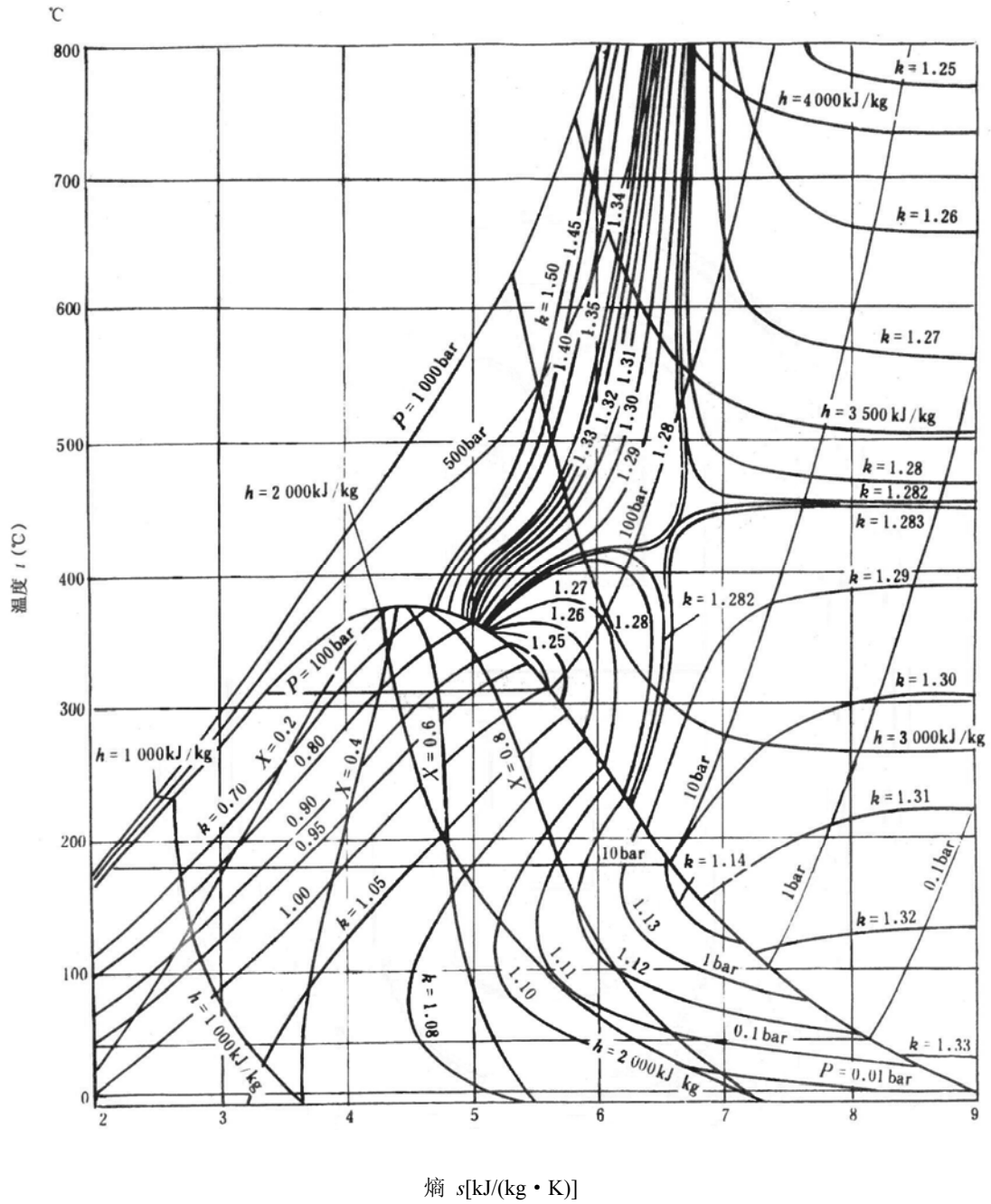
图 B.2 蒸汽绝热指数
